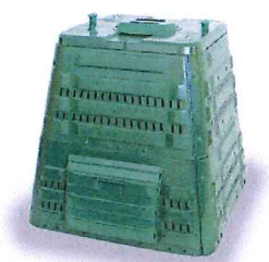
kompostér K400 - objem 400 litrů výška 82 cm rozměry základny 82x82 cm barva zelená hmotnost 12,5 kg
