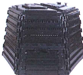
kompostér K900 – objem 950 litrů výška 95 cm průměr základny 150 cm barva zelená hmotnost 29 kg
